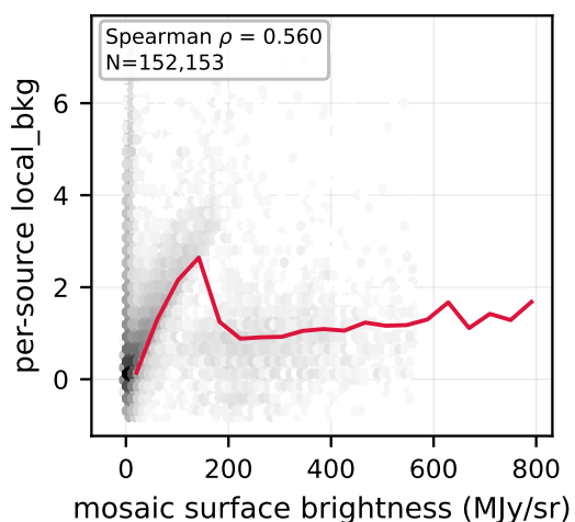
F277W: vs mosaic
