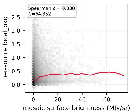
F277W: vs mosaic
